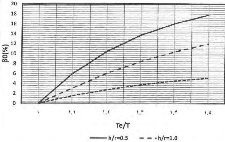
شکل پ-۵-۱ نسبت میرایی پی
