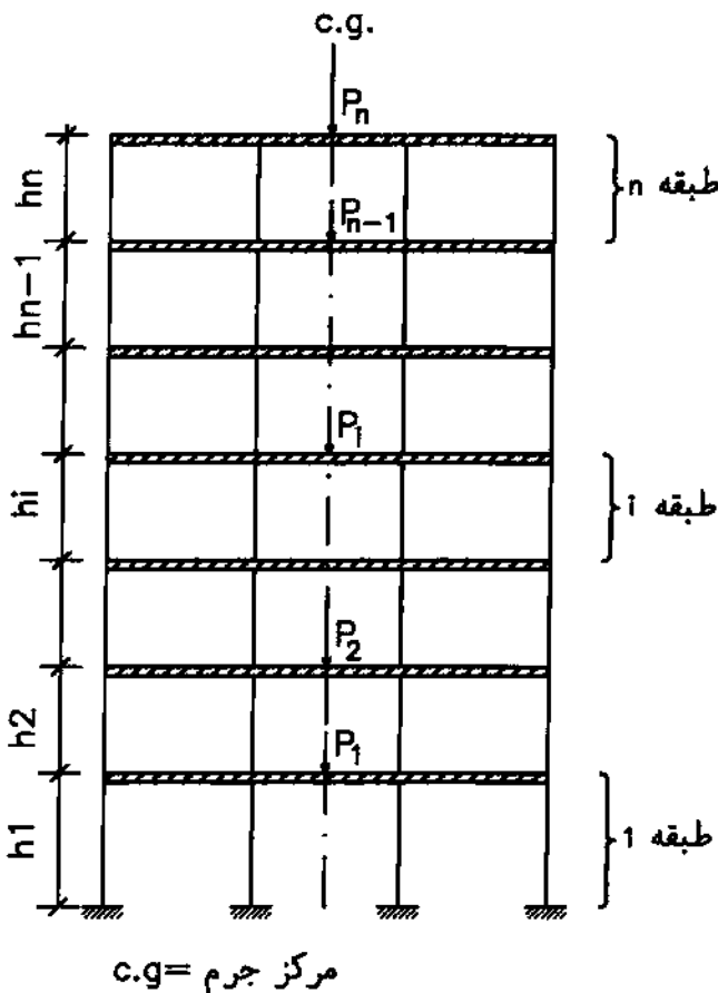
شکل پ-۱ تا پ-۳ سازه چند طبقه تحت اثر بارهای قائم
