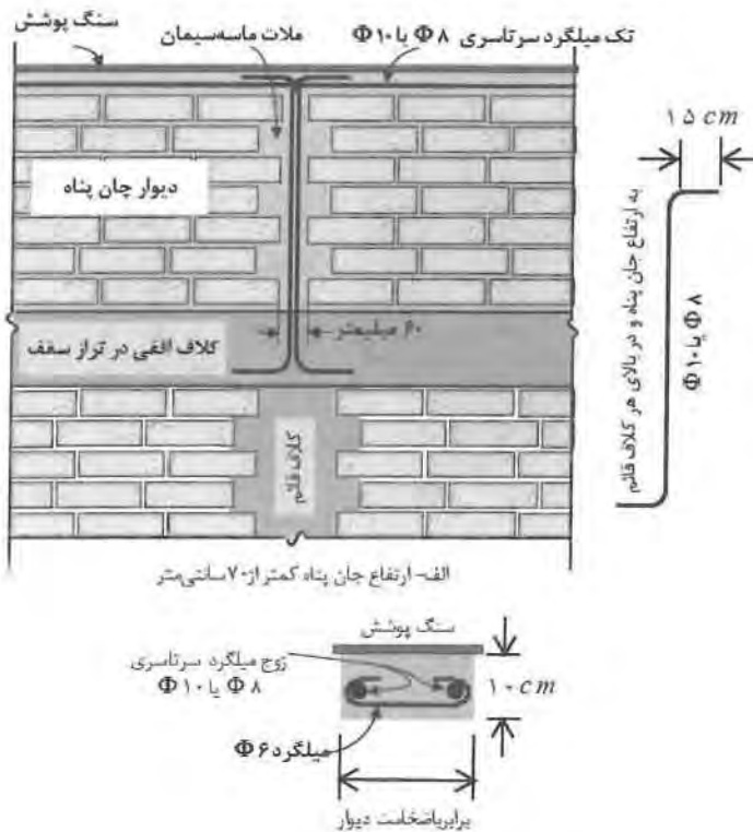
شکل ۷-۱۶ جزئیات مهار جان‌پناه
